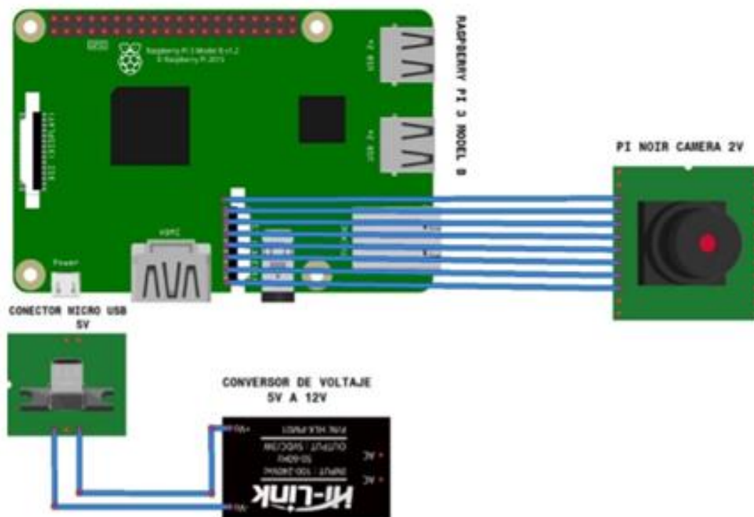
Figura 4. Circuito del sistema propuesto.
